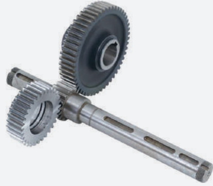
ŞANZUMAN DİŞLİSİ GRUBU Z51-Z31-Z17
