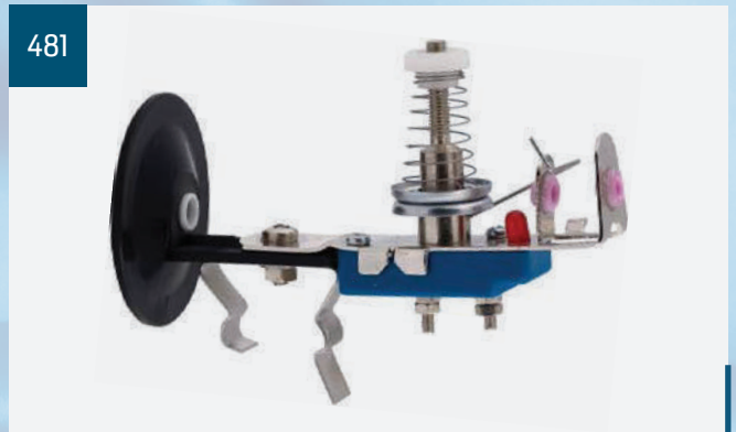
ÇARDAK KONTAĞI
