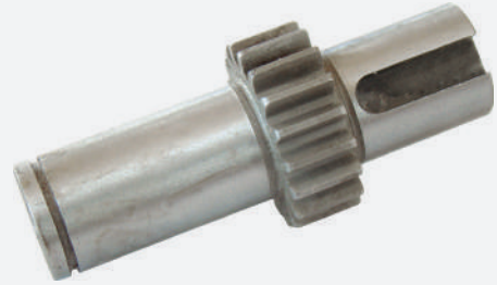
ALT ÇEKTİRME DİŞLİSİ Z16
