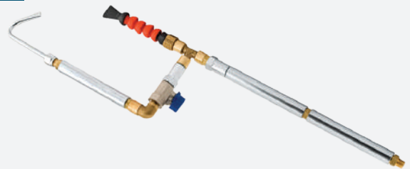
PİLOTELLİ GÖBEK HAVA BORUSU
