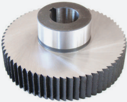
ALT ÇEKTİRME TIRNAK DİŞLİSİ SOL
